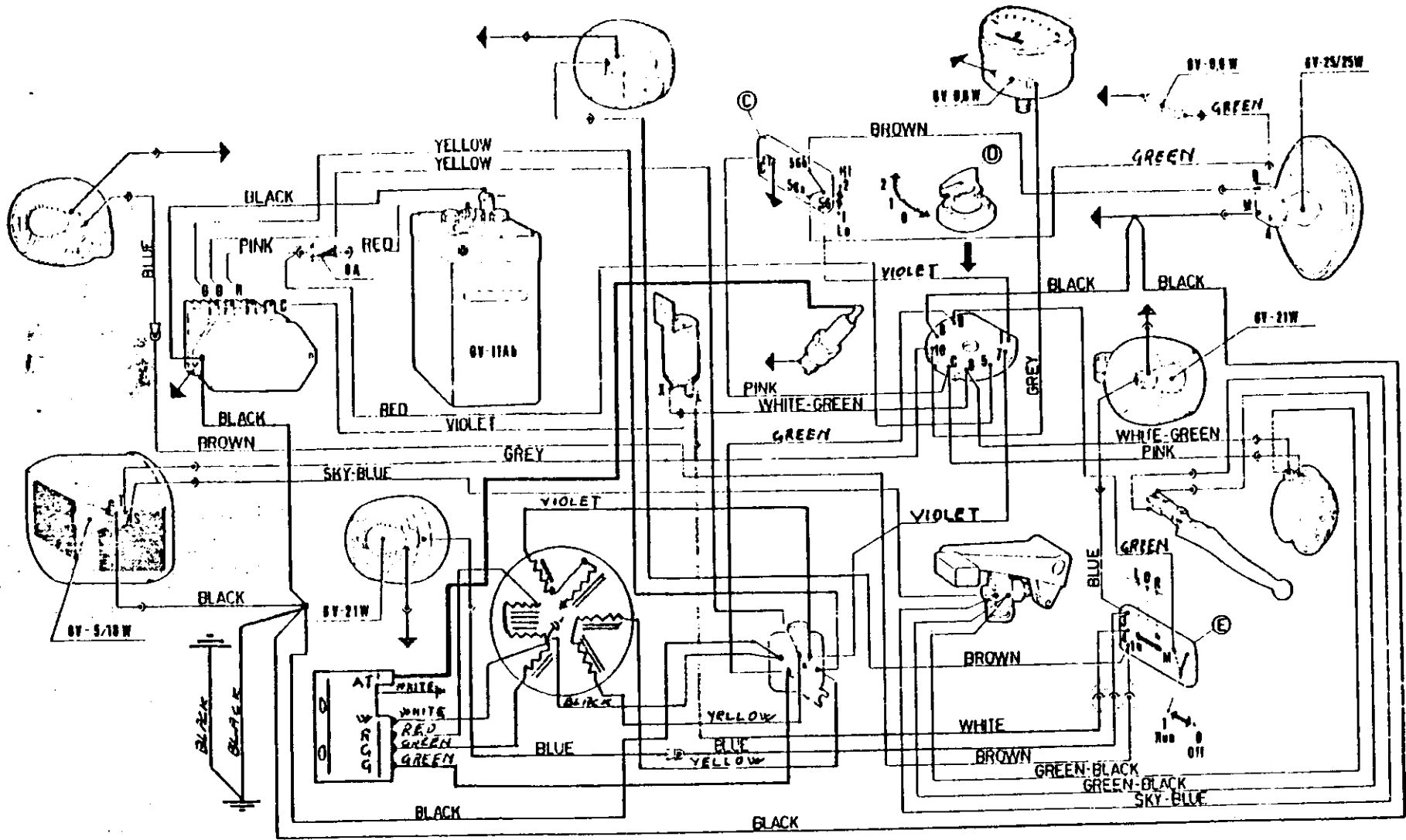
Fig. 1 - Wiring diagram
